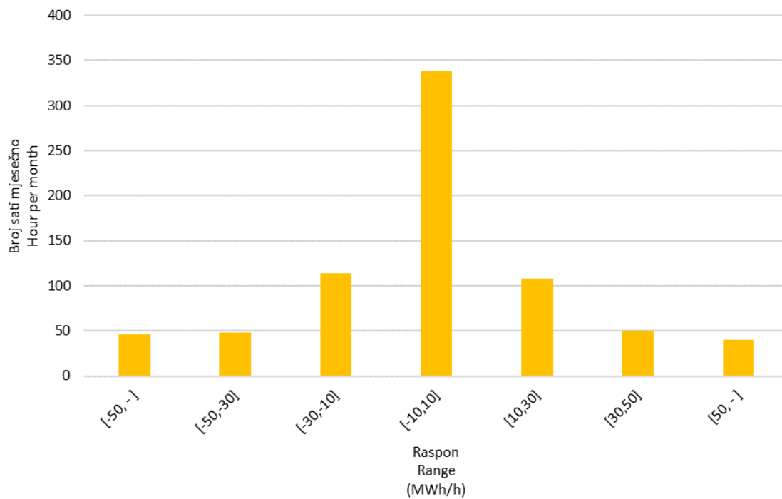
Slika 10 Statistička raspodjela satnih promjena proizvodnje VE u prosincu 2020. godine
