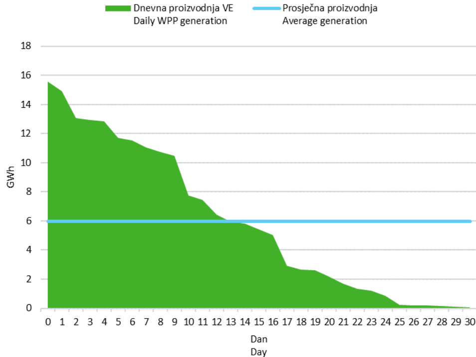
Slika 6 Krivulja trajanja dnevne proizvodnje vjetroelektrana u prosincu 2020. godine
