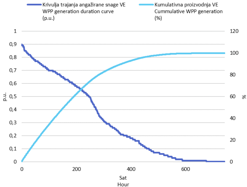
Slika 3 Krivulja trajanja angažirane snage svih VE i kumulativna proizvodnja VE u prosincu 2020. godine u jediničnim vrijednostima
