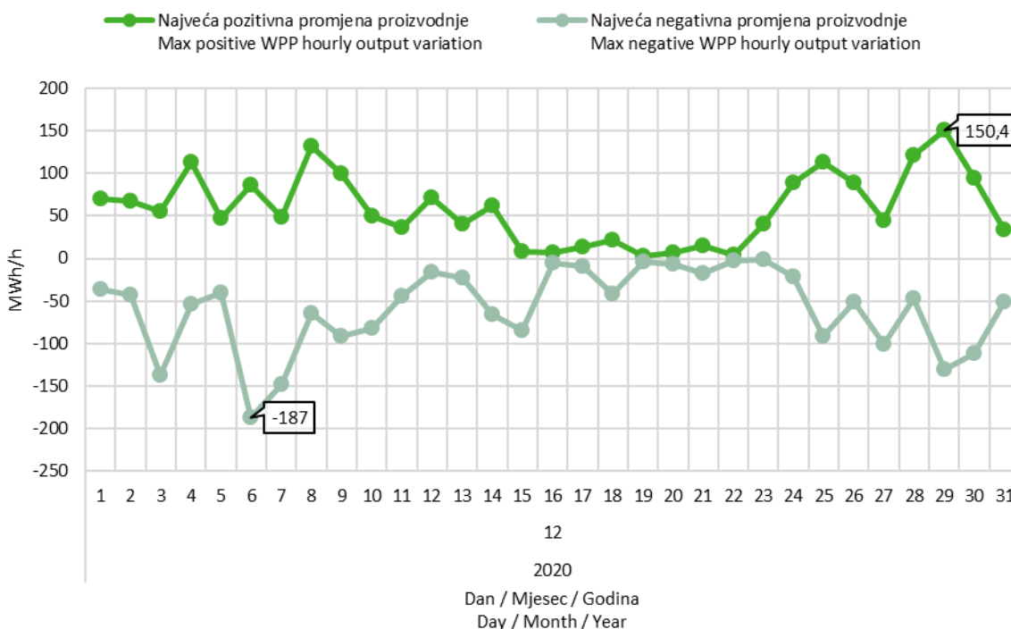
Slika 9 Maksimalna pozitivna i maksimalna negativna promjena satne proizvodnje VE u prosincu 2020. godine
