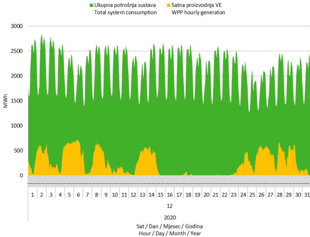
Slika 7 Usporedba satnog dijagrama opterećenja sustava i proizvodnje vjetroelektrana u prosincu 2020. godine
