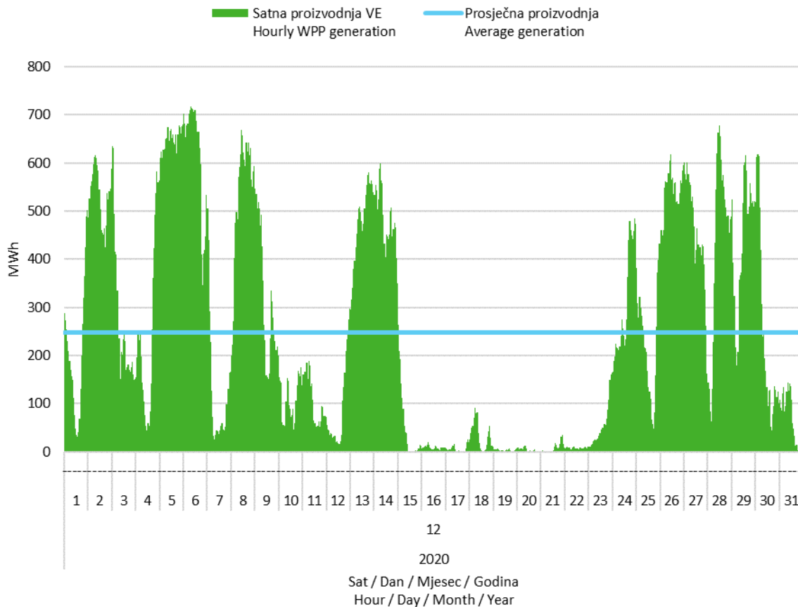
Slika 2 Satna proizvodnja svih vjetroelektrana u prosincu 2020. godine
