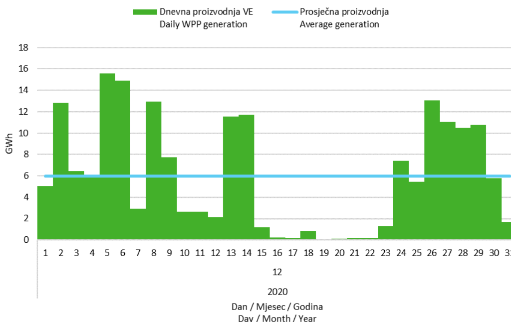
Slika 5 Dnevna proizvodnja svih vjetroelektrana u prosincu 2020. godine
